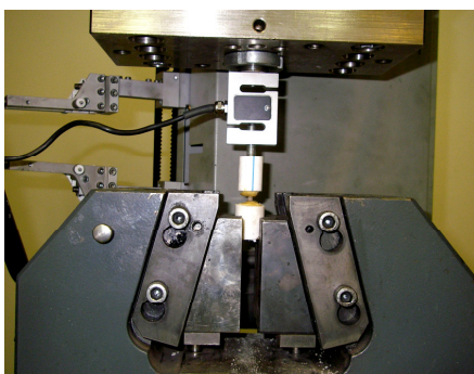
تصویر ۵: نمونه متصل به دستگاه کشش
