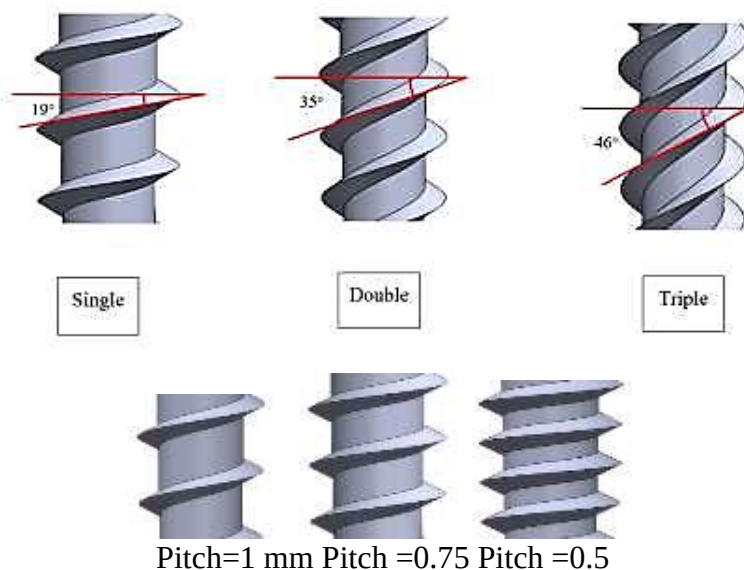
شکل ۱. پارامترهای طراحی رزوه در محیط نرم افزار SolidWorks
