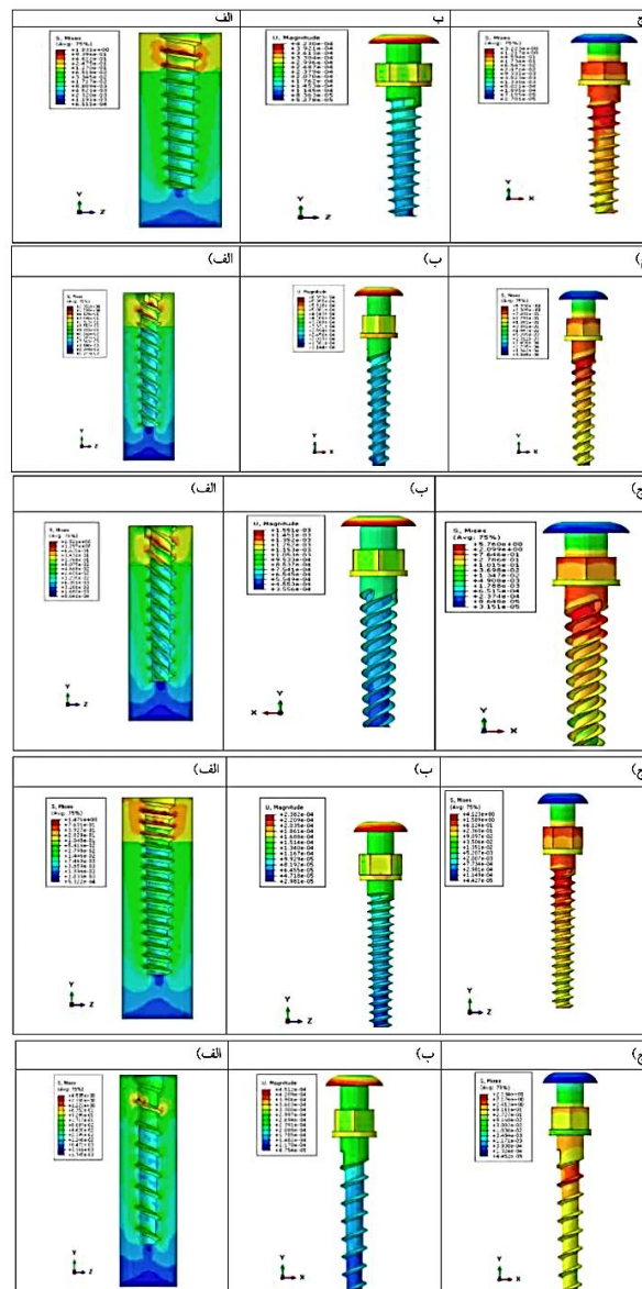
شکل ۳. (الف) توزیع استرس در استخوان (مگاپاسکال) (ب) میزان جابه جایی (میکرومتر) (ج) توزیع استرس در مینی اسکرو (مگاپاسکال) تحت اعمال نیروی کششی در نمای اگزیتال
