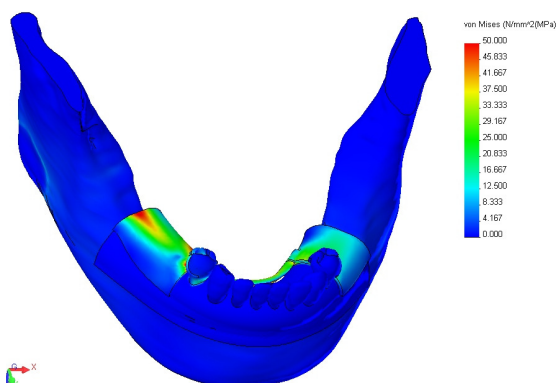
تصویر ۲: نگاره رایانه ای پس از انجام مراحل اعمال نیرو و آنالیز اجزاء محدود
