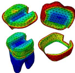
تصویر ۶: توزیع دما در بخش‌های مختلف دندان ترمیم شده با سرامیک در اثر اعمال تحریک گرم
