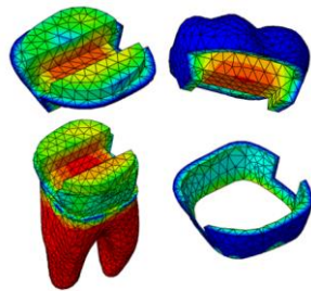
تصویر ۴: توزیع دما در بخش‌های مختلف دندان ترمیم شده با سرامیک در اثر اعمال تحریک سرد
