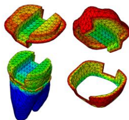
تصویر ۷: توزیع دما در بخش‌های مختلف دندان ترمیم شده با طلا در اثر اعمال تحریک گرم
