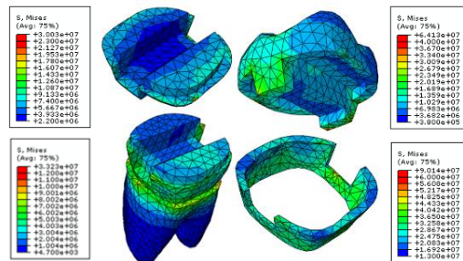
تصویر ۸: توزیع تنش در بخش‌های مختلف دندان ترمیم شده با سرامیک در اثر اعمال تحریک سرد
